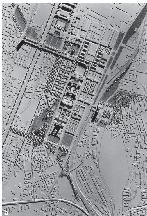
Fig. 7.4 Due approcci diversi allo stesso problema urbano: il concorso per l'area ex Pirelli Bicocca a Milano (1985-88). a) La proposta presentata da Gregotti Associati si pone in continuità con lo schema urbano circostante, enfatizzandolo. Fonte: AA.VV., Progetto Bicocca , Electa 1986 © Gregotti Associati. b) Quella di Roberto Gabetti e Aimaro Isola si appoggia provocatoriamente sull'antico orientamento dell'organizzazione romana del territorio, obliterata dagli sviluppi successivi, dando luogo a situazioni inedite e non prevedibili. Fonte: Archivio Gabetti e Isola.
