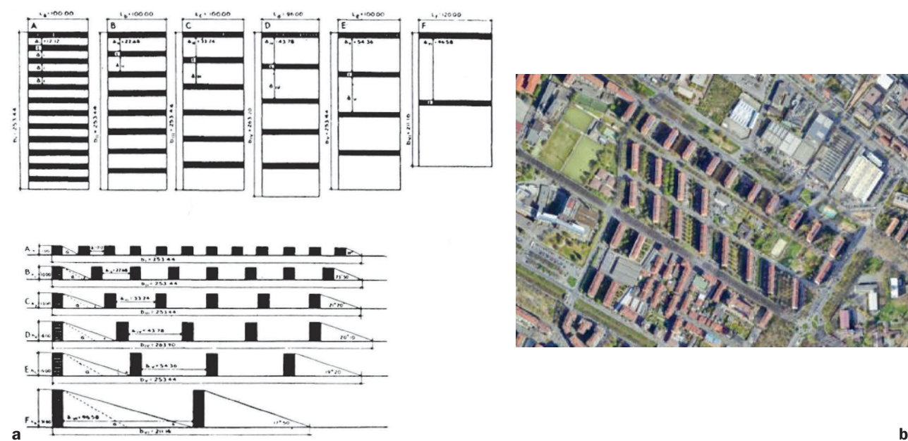
Fig. 7.3 a) Walter Gropius, possibili sviluppi di un'area edificabile con edifici di diversa altezza, da Costruzioni basse, medie o alte? , intervento al III CIAM, Metodi costruttivi razionali, Bruxelles 1930. b) Porzione di tessuto urbano costituito da edifici con orientamento prossimo all'asse elioterminico (Torino): la relazione con la trama viaria è questionabile. Fonte: Google Maps.
